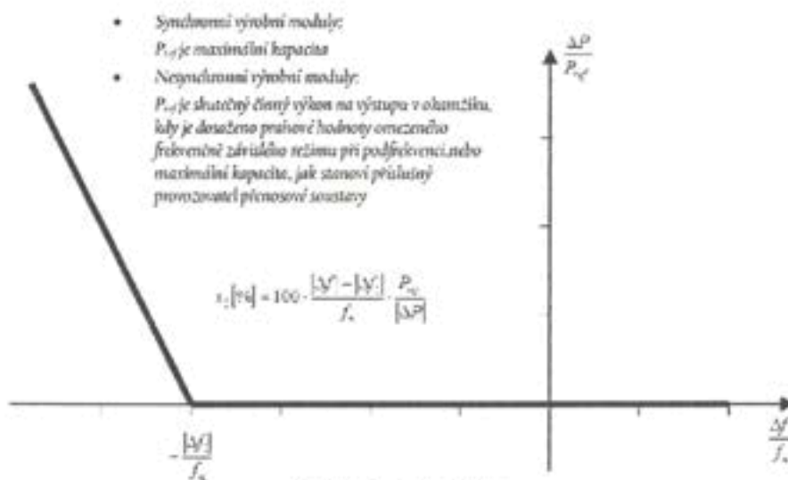
Obr. 3 Diagram LFSM-U
