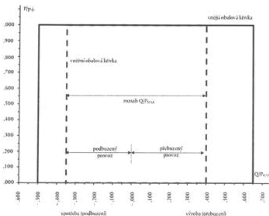
Profil P-Q/P_{max} nesynchronního výrobního modulu.
