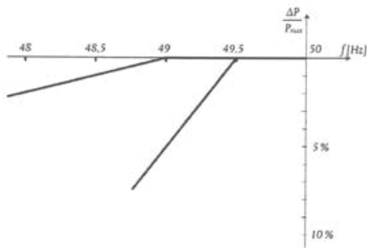
Obr. 2 Připustné snížení činného výkonu s klesající frekvencí
