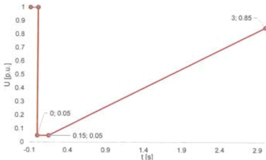
Obr. 11 Časovým průběhem napětí v místě připojení za podmínek poruchy pro nesynchronní výrobní moduly kategorie A, B a C (FRT křivka)
