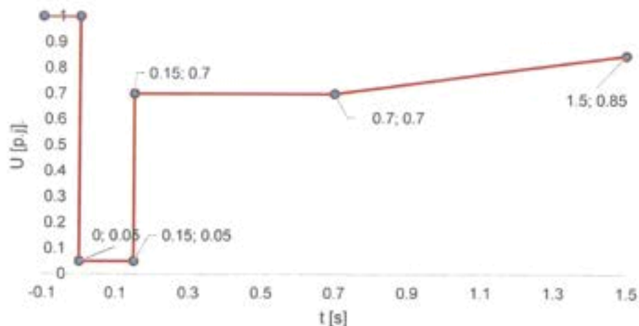
Obr. 10 Časovým průběhem napětí v místě připojení za podmínek poruchy pro synchronní výrobní moduly od 1MW - kategorie B2 a C (FRT křivka)
