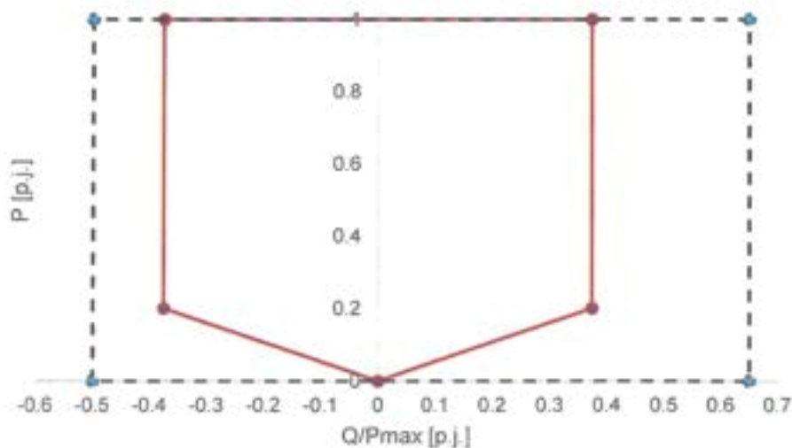
Obr. 8 Diagram dodávky jalového výkonu při nižší než maximální dodávce činného výkonu pro nesynchronní výrobní moduly kategorie D
