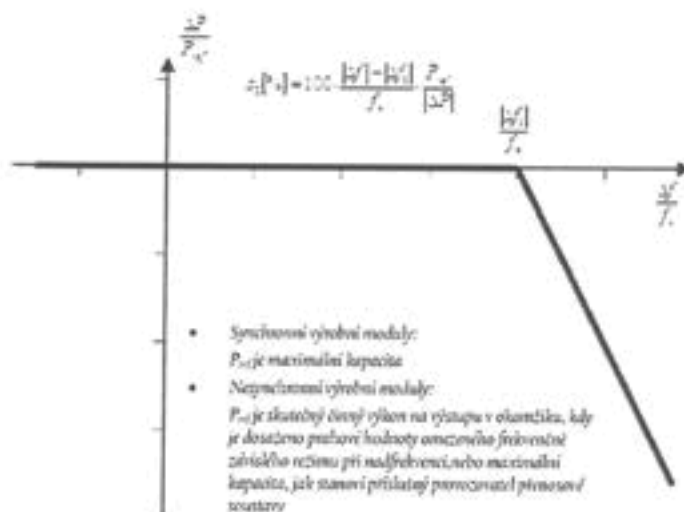
Obr. 1 Diagram LFSM-O
