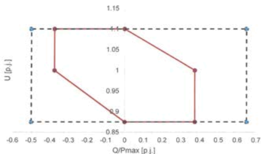
Obr. 7 Diagram dodávky jalového výkonu při maximální dodávce činného výkonu pro nesynchronní výrobní moduly kategorie D
