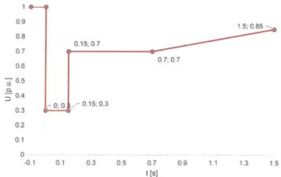
Obr. 9 Časovým průběhem napětí v místě připojení za podmínek poruchy pro synchronní výrobní moduly do 1MW - kategorie A1, A2, B1 (FRT křivka)
